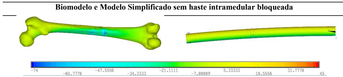
Fig. 6. Tensões normais em flexão plana nos modelos sem haste, MPa.
